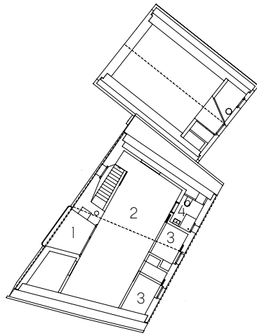
Grundriss DG
