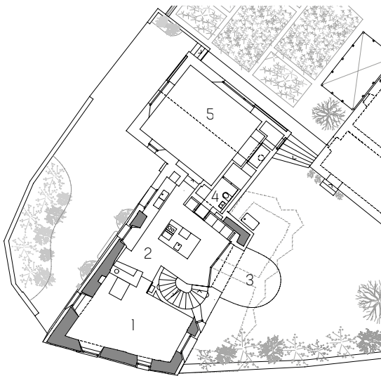
Grundriss 1. OG
